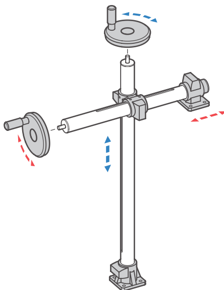
Einrohr-Verstelleinheiten Kombination mit Verstellung in X- / Z-Richtung
