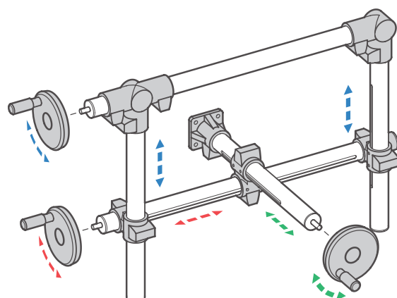
Portalaufbau mit Verstellung in Z- / X- / Y-Richtung
